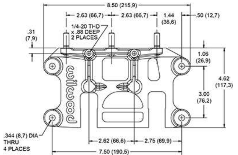
VIEW A-A
